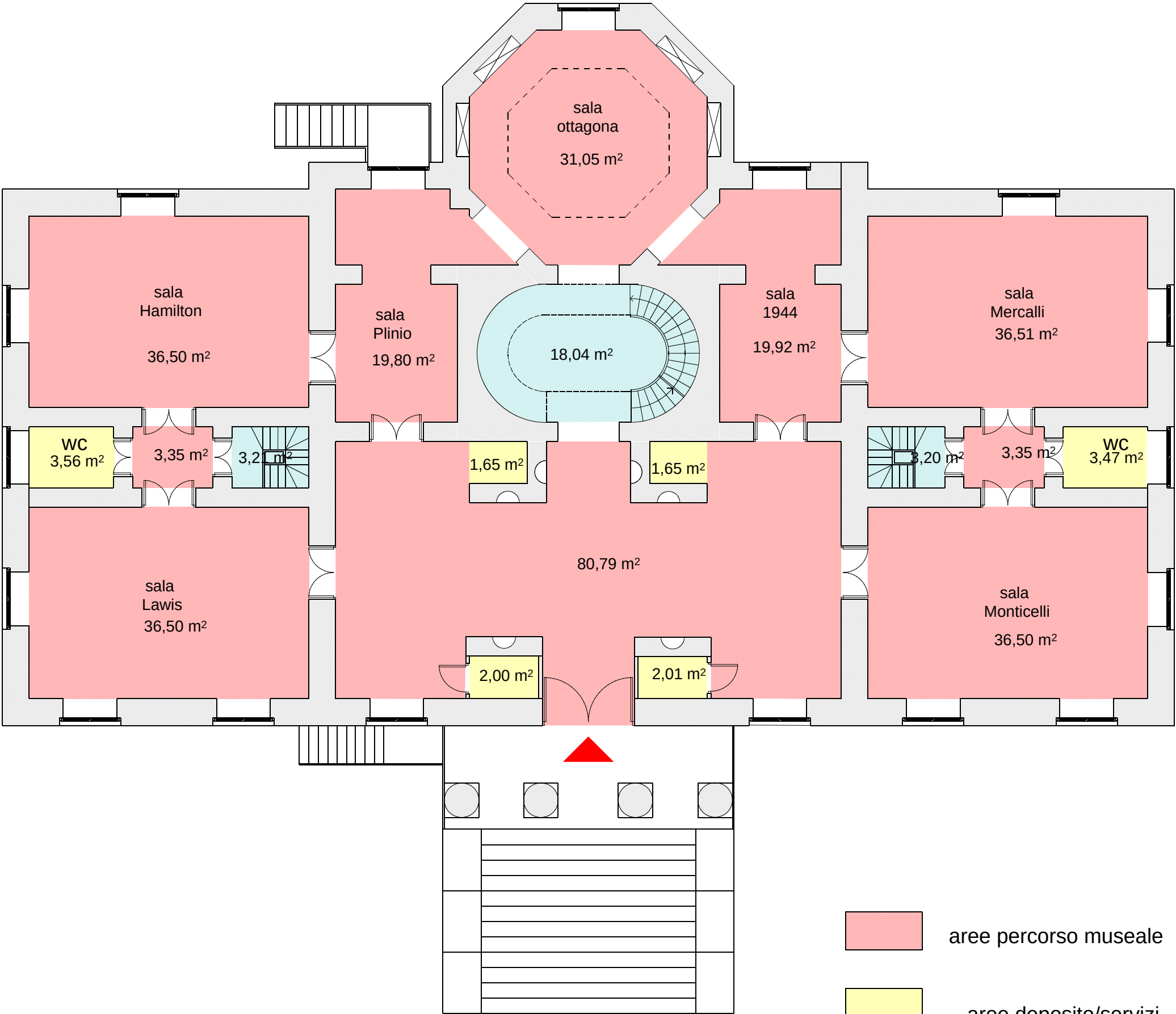
EDIFICIO STORICO sede di Ercolano Pianta piano rialzato
